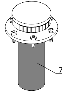
BOUCHON DE REMPLISSAGE COMPLET KOMPLETTER EINFÜLLVERSCHLUSS TAPON DE LLENADO COMPLETO COMPLETE FILLING PLUG TAPPO DI RIEMPIMENTO COMPLETO
