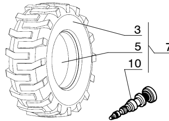
OTR TREAD 802674 (2WD)
